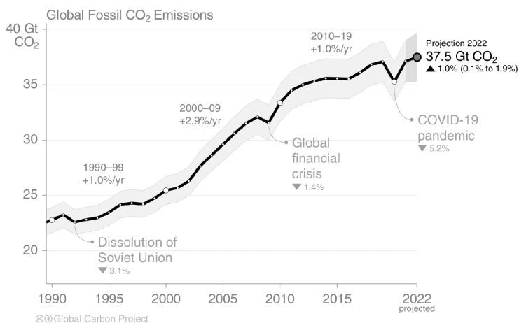
Abb 1: Entwicklung der globalen Treibhausgas-Emissionen 1990–2022 [Global Carbon Project, 2023, https://robbieandrew.github.io/GCB2022/PNG/s11_2022_FossilFuel_and_Cement_emissions_1990.png (18.11.2023)]
