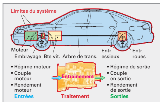
Illustration 3 : Sous-système : entraînement
